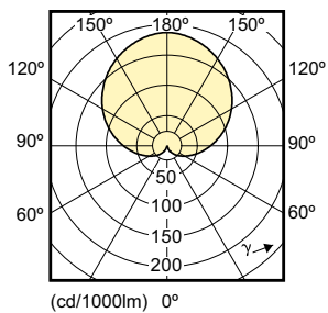
A60/ A67 E27 FR
