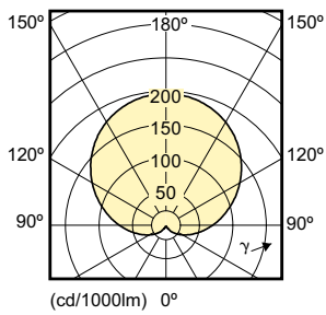
5.5-40W E27 A60 WW 2700 K
