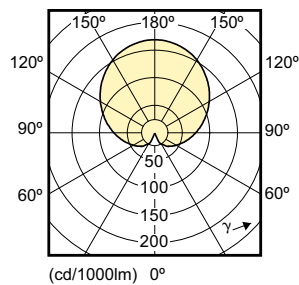
5.5-40W A60 E27 /865
