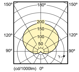
11.5-75W E27 827 2700K A67
