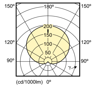
100W E27 A60
