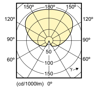
13.5-100 W, 9-60 W E27 G93 /827 FR
