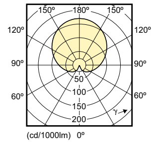
6-40W A60 E27 /830
