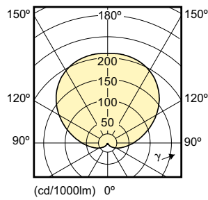
15-100 W E27 A67 /827 2700 K
