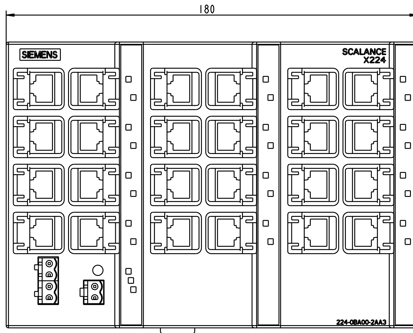
Vorne / Front
