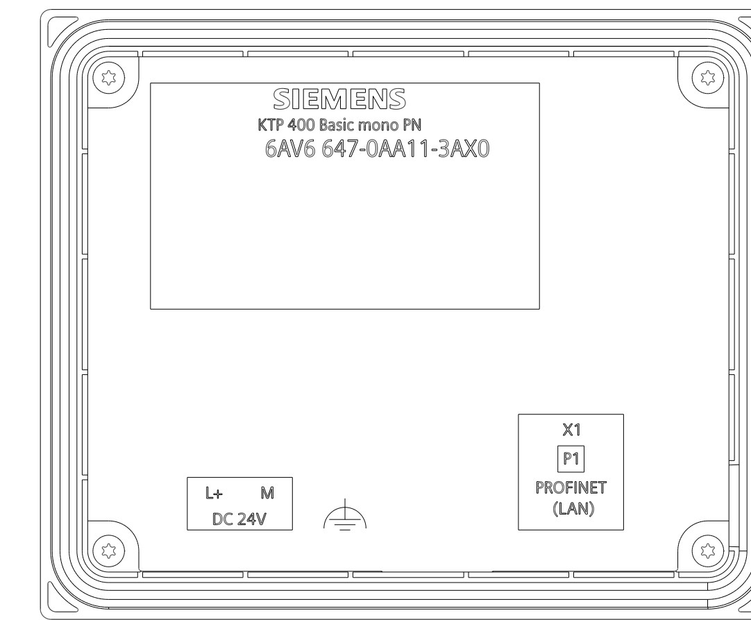
Hinten / Back
