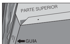
Figura 1 La cara de la cámara de pared debe sobresalir entre ½ y 5/8 de pulgada de la cara del puntal a fin de dejar espacio para la lámina de yeso.
