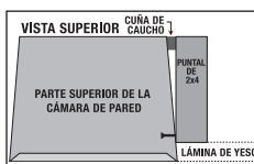
Figura 2 Conecte la cámara de pared al puntal mediante los tornillos. (Aparece el modelo CS)
